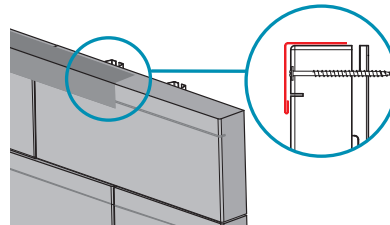
HAUT DE MUR + RANG PERCÉ AVEC MOULURE DE FINITION FIGURE 10
