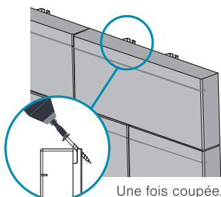
EN MILIEU DE MUR FIGURE 8
