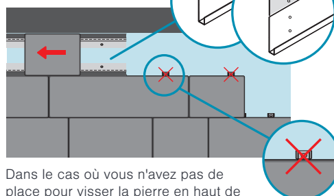
HAUT DE MUR AVEC MOULURES EN J FIGURE 9
