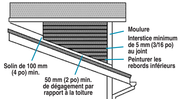
FIGURE 2 VUE DÉTAILLÉE D'UN SOLIN DE TOIT
